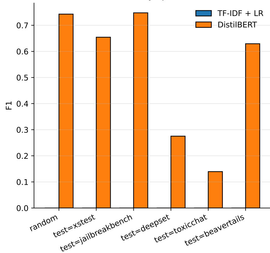
F1 by split
