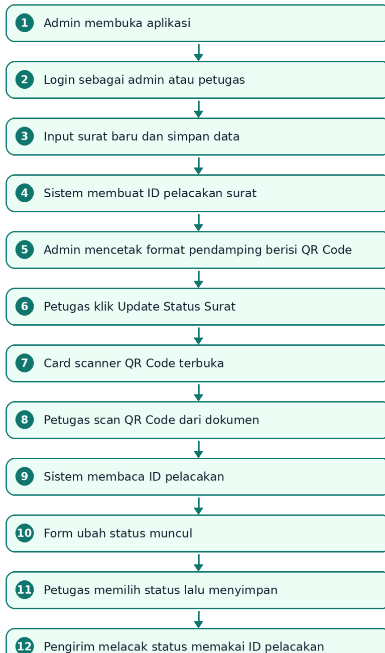
Gambar 1. Alur kerja utama aplikasi TUS Tracking Surat
