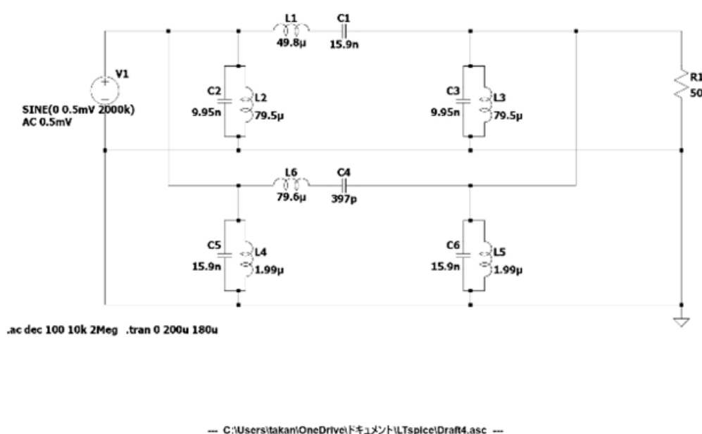
図 70: マルチバンドパスフィルタの回路図
