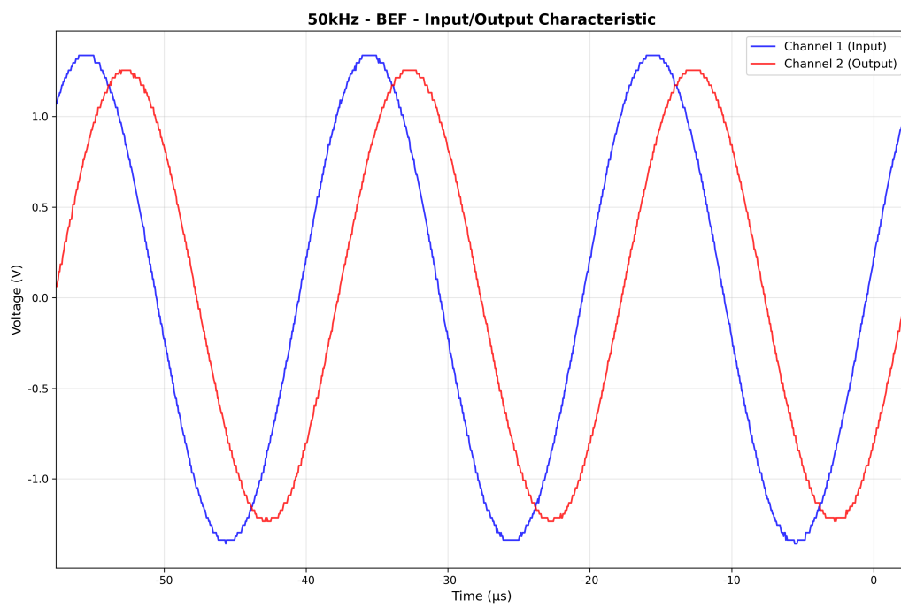
图 54: 50kHz BEF 波形
