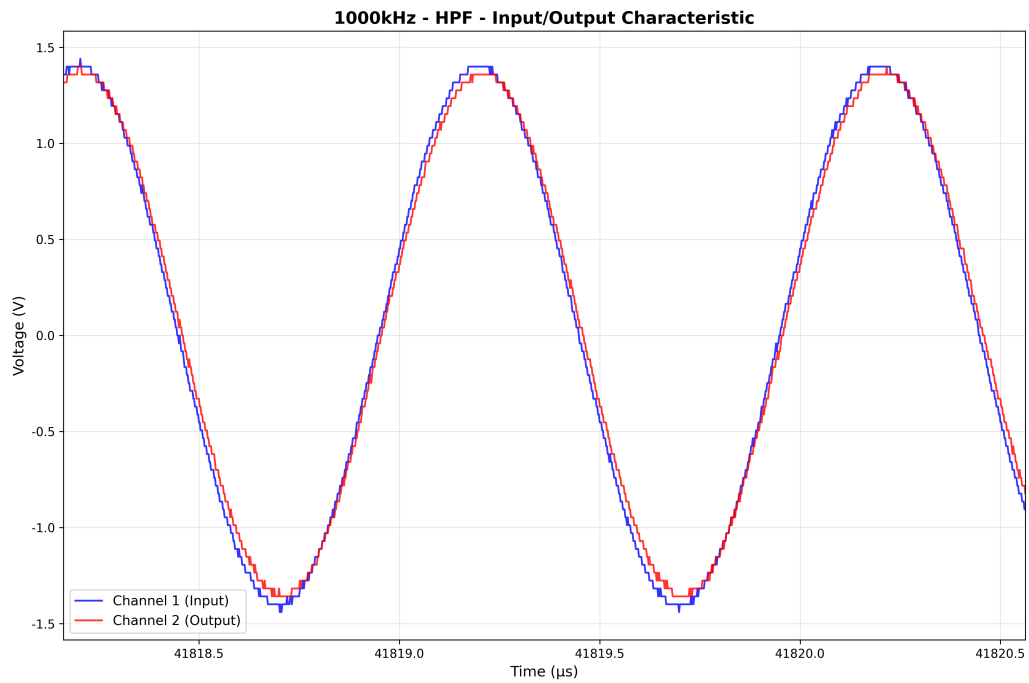
図 31: 1000kHz HPF 波形
