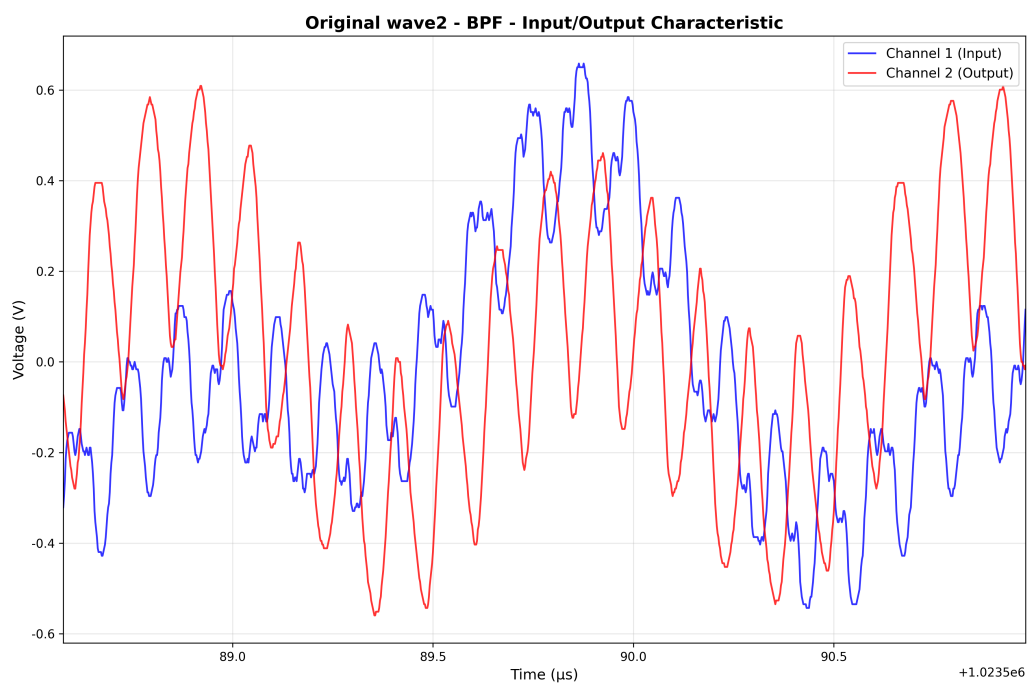
图 48: Original wave2 BPF 波形
