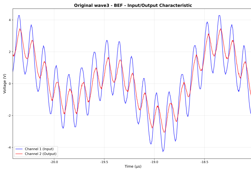
图 64: Original wave3 BEF 波形
