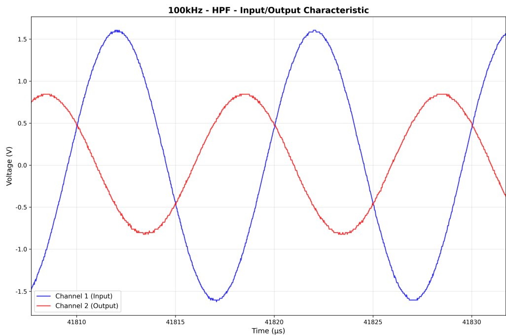
图 27: 100kHz HPF 波形
