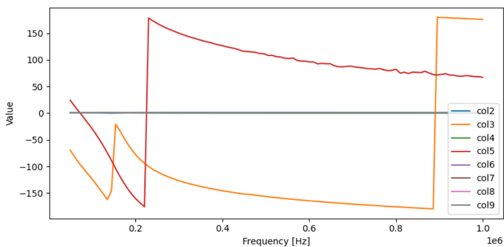
図 68: BPF の周波数特性 (NanoVNA 測定)
