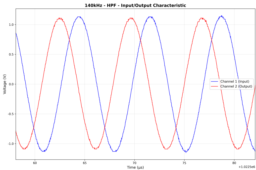
图 28: 140kHz HPF 波形
