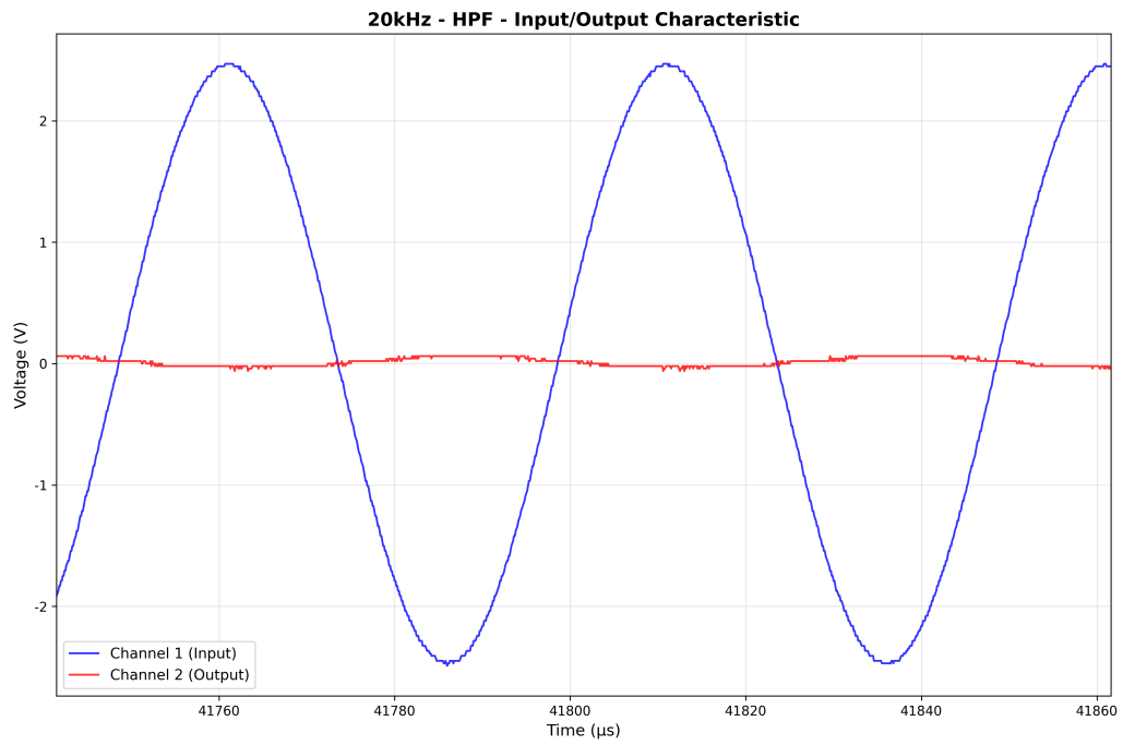
图 23: 20kHz HPF 波形
