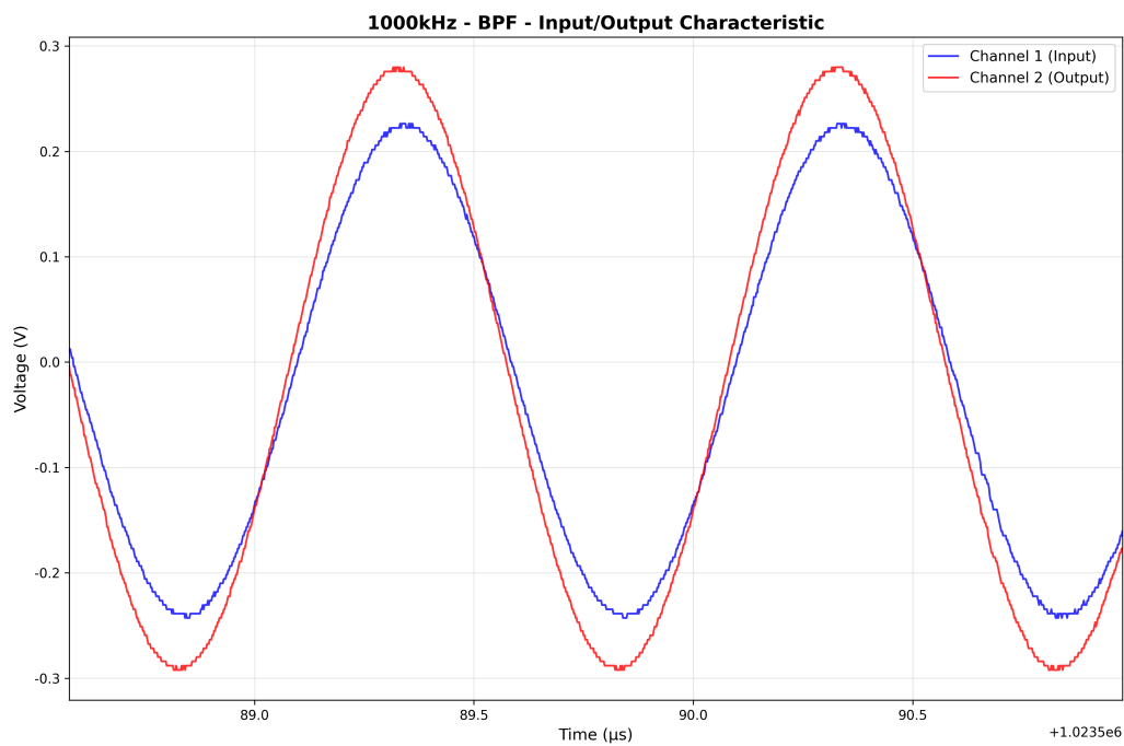
図 45: 1000kHz BPF 波形
