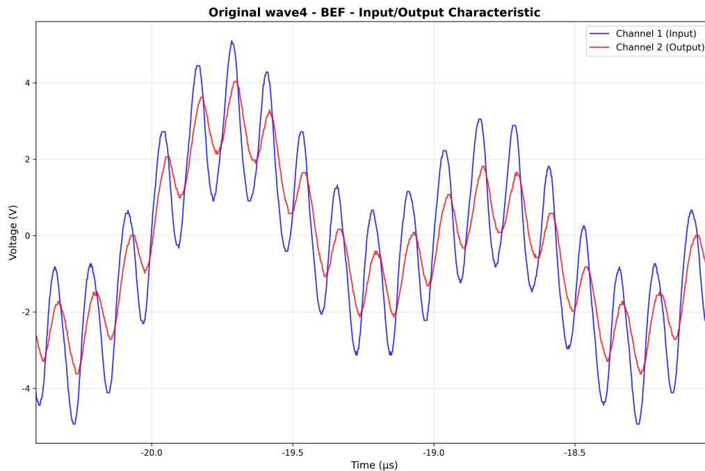
図 65: Original wave4 BEF 波形
