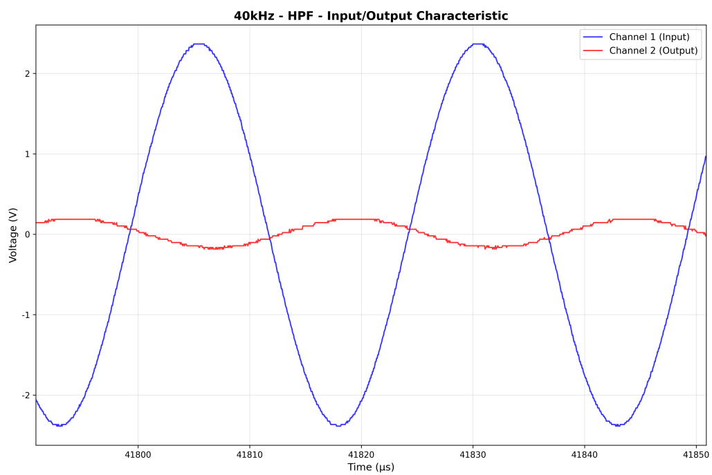
图 24: 40kHz HPF 波形
