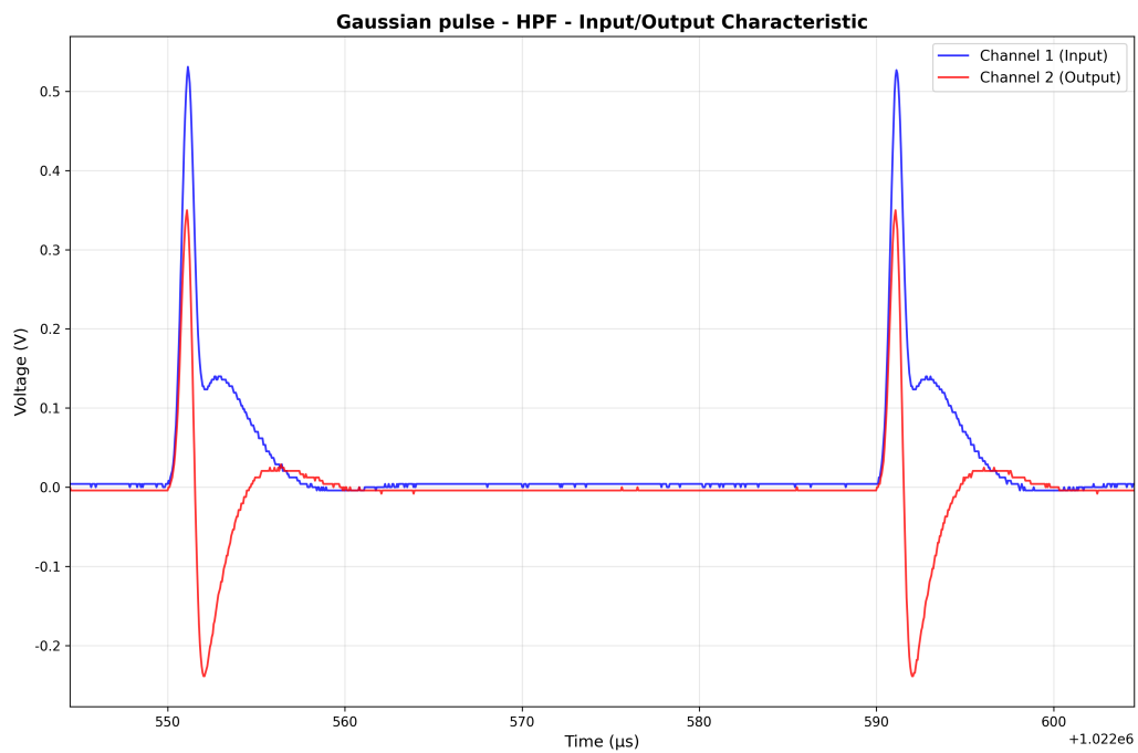
図 32: HPF の出力波形 (ガウシアンパルス)
