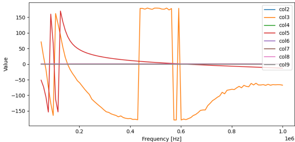
図 69: BEF の周波数特性 (NanoVNA 測定)
