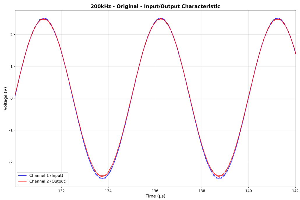
图 14: 200kHz LPF 波形
