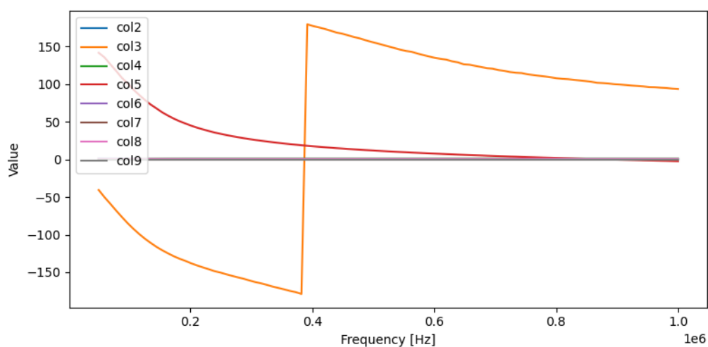
図 67: HPF の周波数特性 (NanoVNA 測定)
