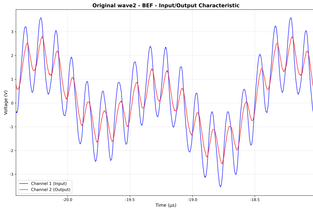
图 63: Original wave2 BEF 波形
