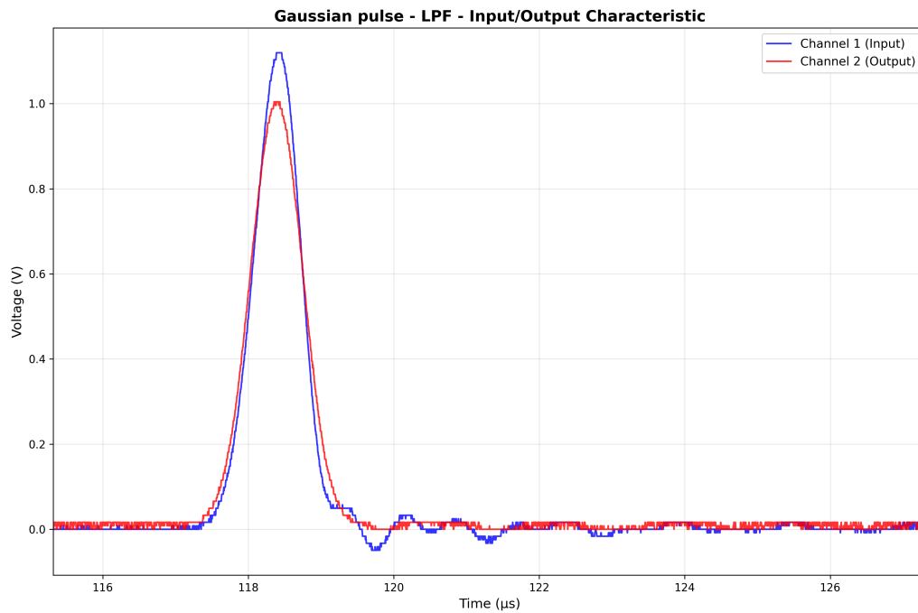
図 17: LPF の出力波形 (ガウシアンパルス)
