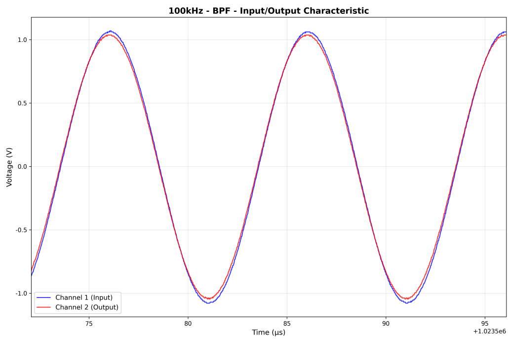
图 42: 100kHz BPF 波形
