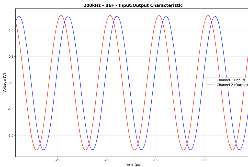
图 58: 200kHz BEF 波形
