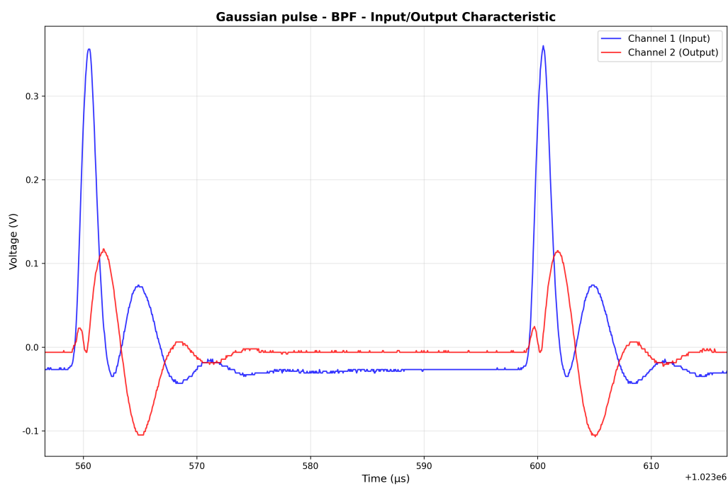
図 46: BPF の出力波形 (ガウシアンパルス)
