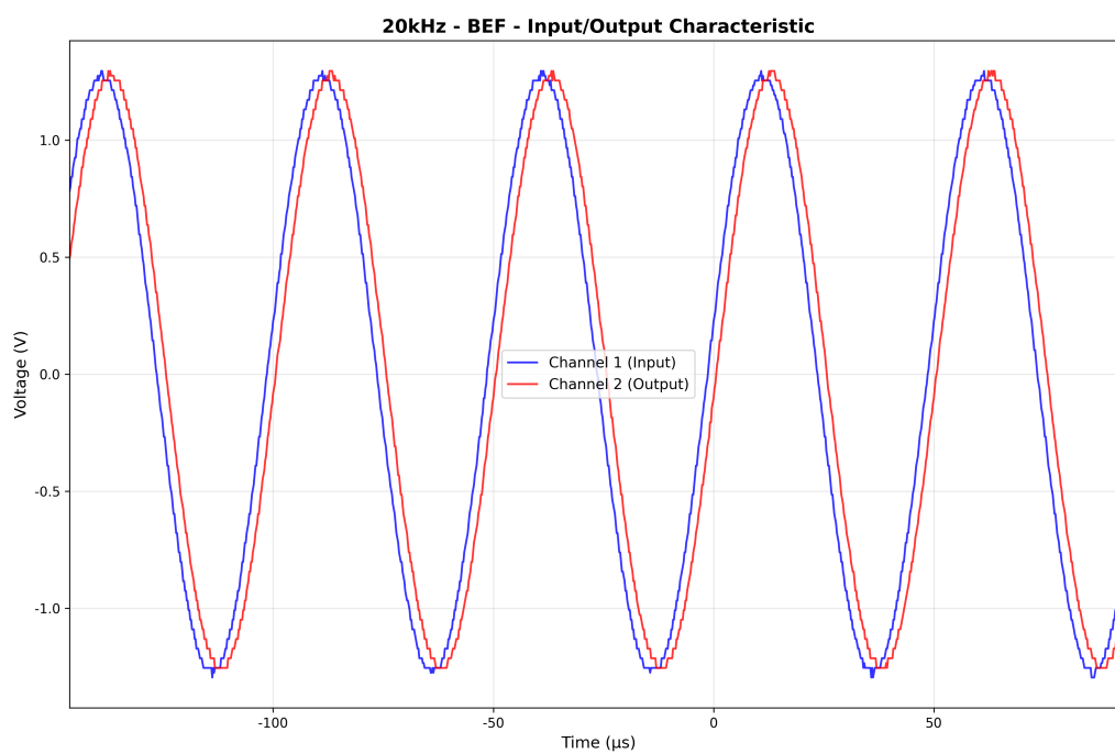
图 52: 20kHz BEF 波形
