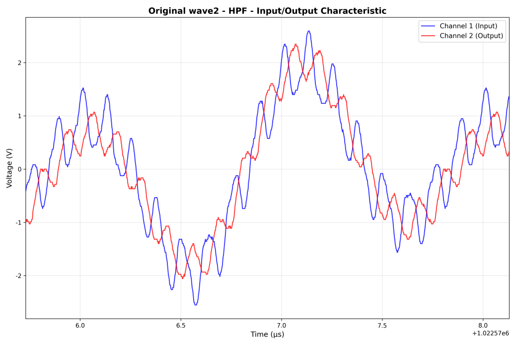
图 34: Original wave2 HPF 波形
