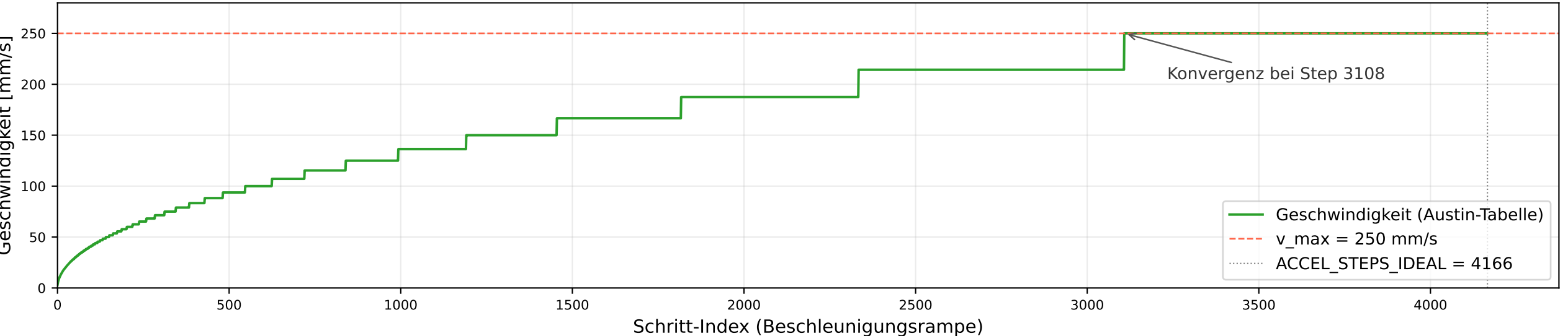
Austin-Formel Ramp-Table — Beschleunigungsrampe (X/Y-Achsen)
