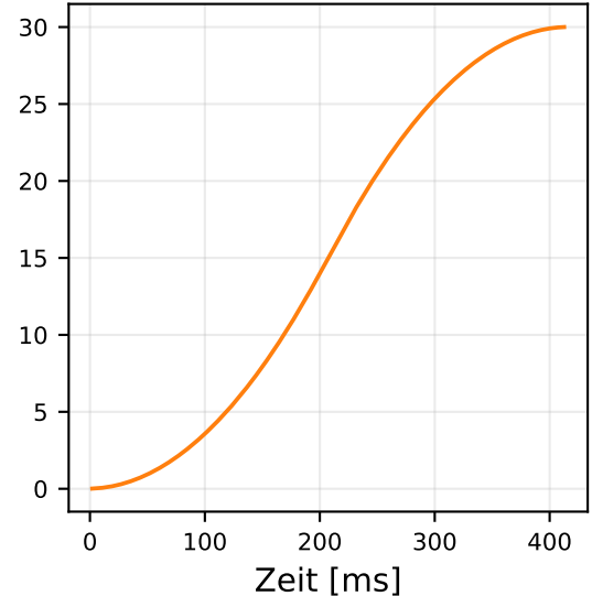
Austin-Formel Ramp-Table — Beschleunigungsrampe (X/Y-Achsen)
