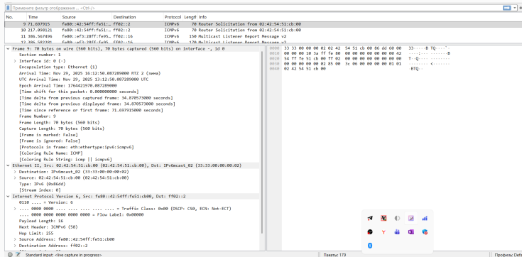
Рис. 43: анализ трафика
