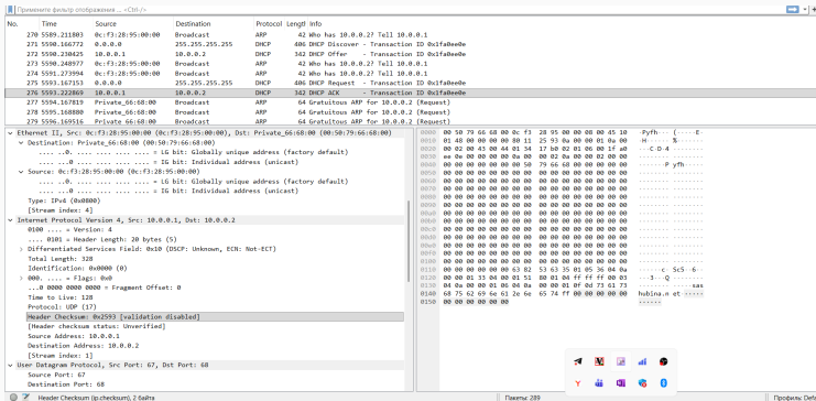
Рис. 24: анализ трафика
