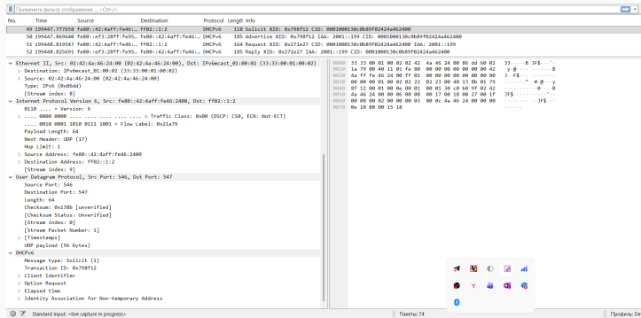
Рис. 54: анализ трафика
