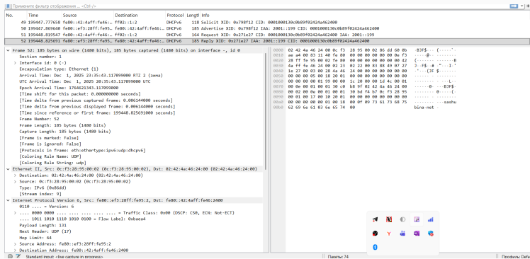
Рис. 59: анализ трафика
