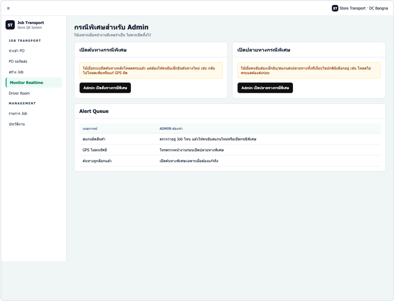
หน้าจำลองปุ่มเปิดต้นทาง/ปลายทางกรณีพิเศษ และ Alert Queue
