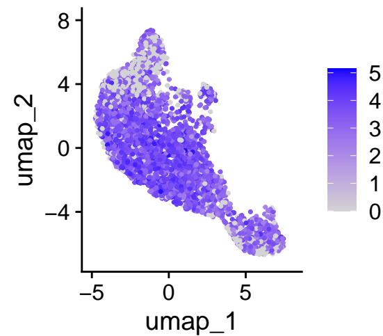
GUK1
