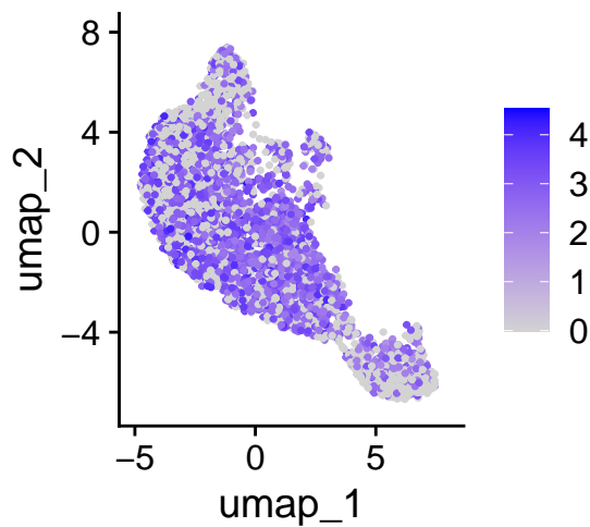
DSC2
