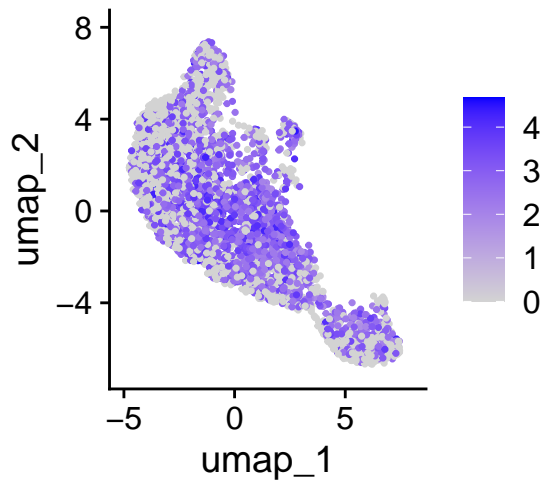
DSC2
