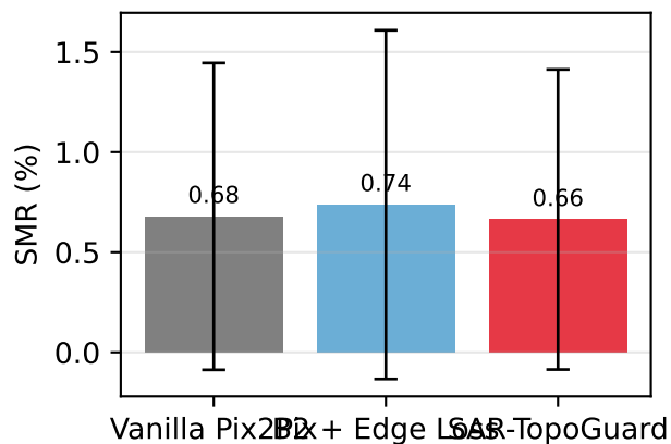
(d) SMR
