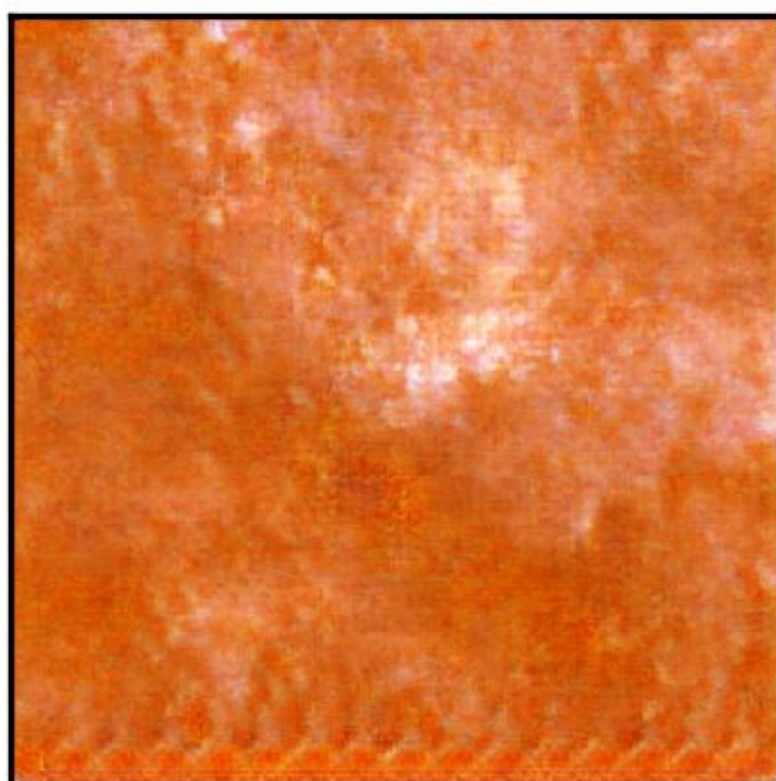
SAR-TopoGuard
