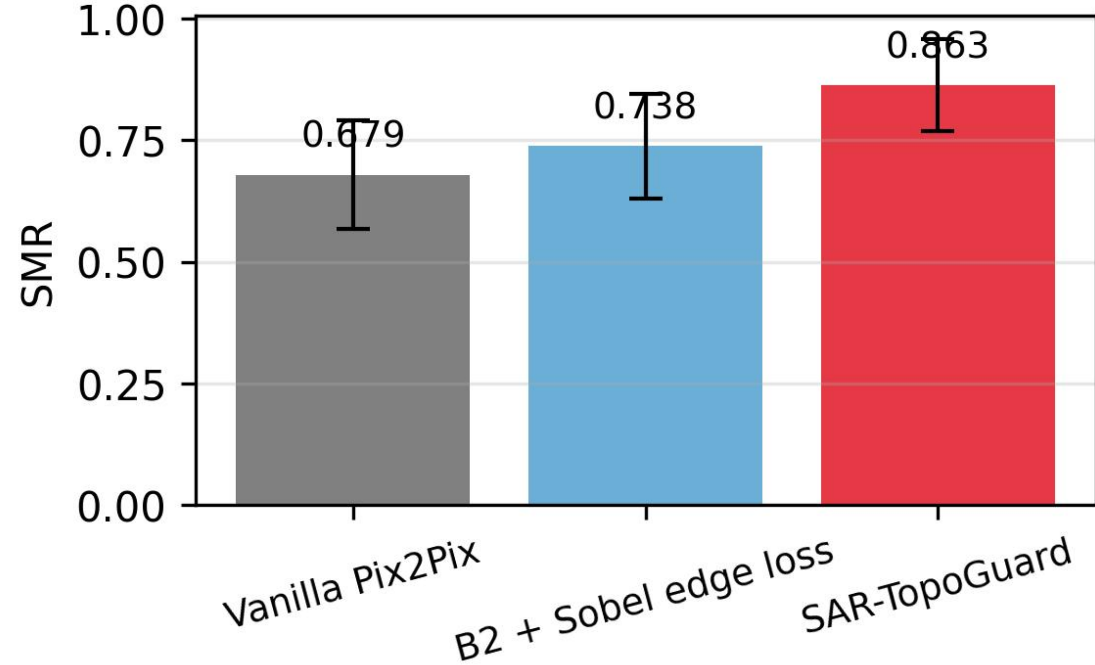
(d) SMR
