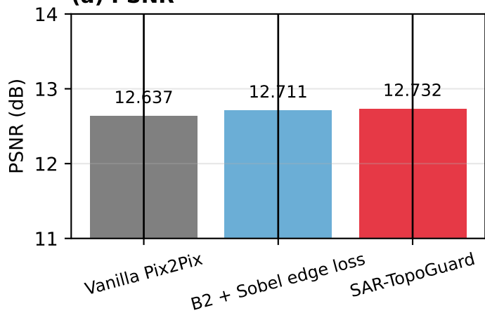
(a) PSNR
