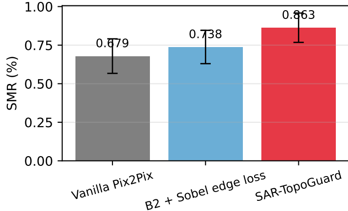
(d) SMR
