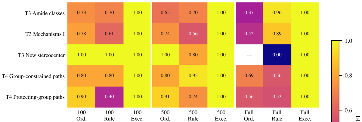
Qwen3.5-397B-A17B
