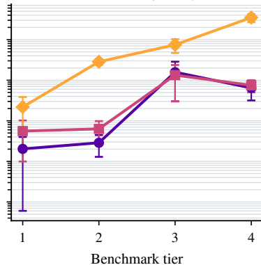
(d) Tool time (s) / trajectory
