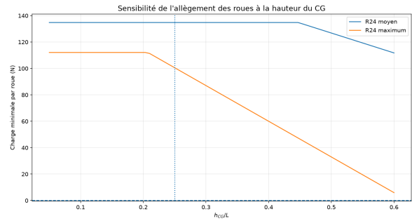
(b) Sensibilité de l'allègement des roues à la hauteur du centre de gravité.
