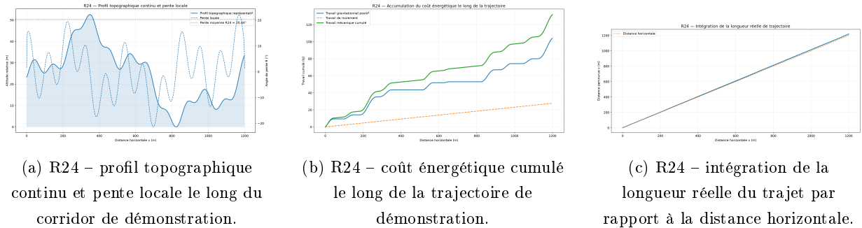
Figure 18: Profil topographique continu et pente locale le long du corridor de démonstration (a) ; coût énergétique cumulé (b) ; intégration de la longueur réelle du trajet (c).
