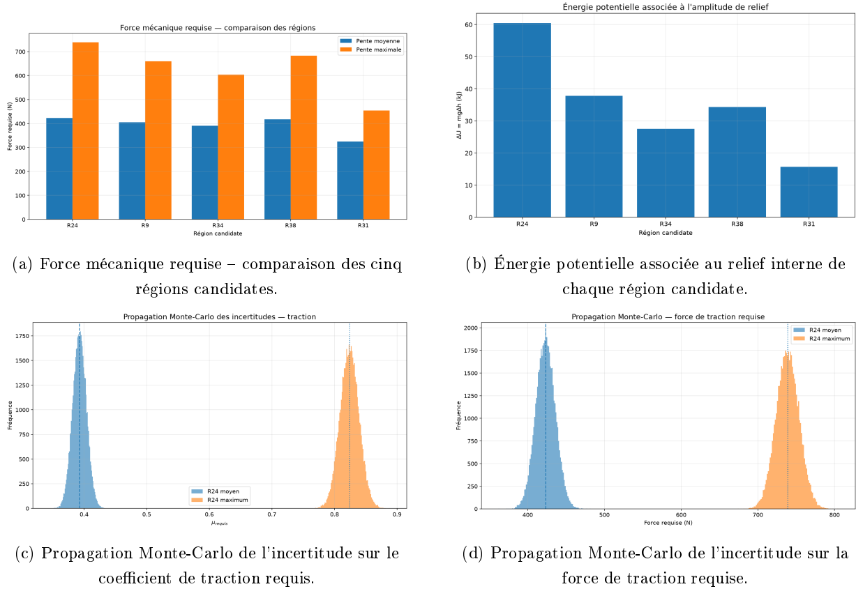
Figure 34: Force mécanique requise selon les candidats (a) ; énergie potentielle issue du relief interne (b) ; propagation Monte-Carlo de l'incertitude sur \mu_{req} (c) et sur la force de traction requise (d).
