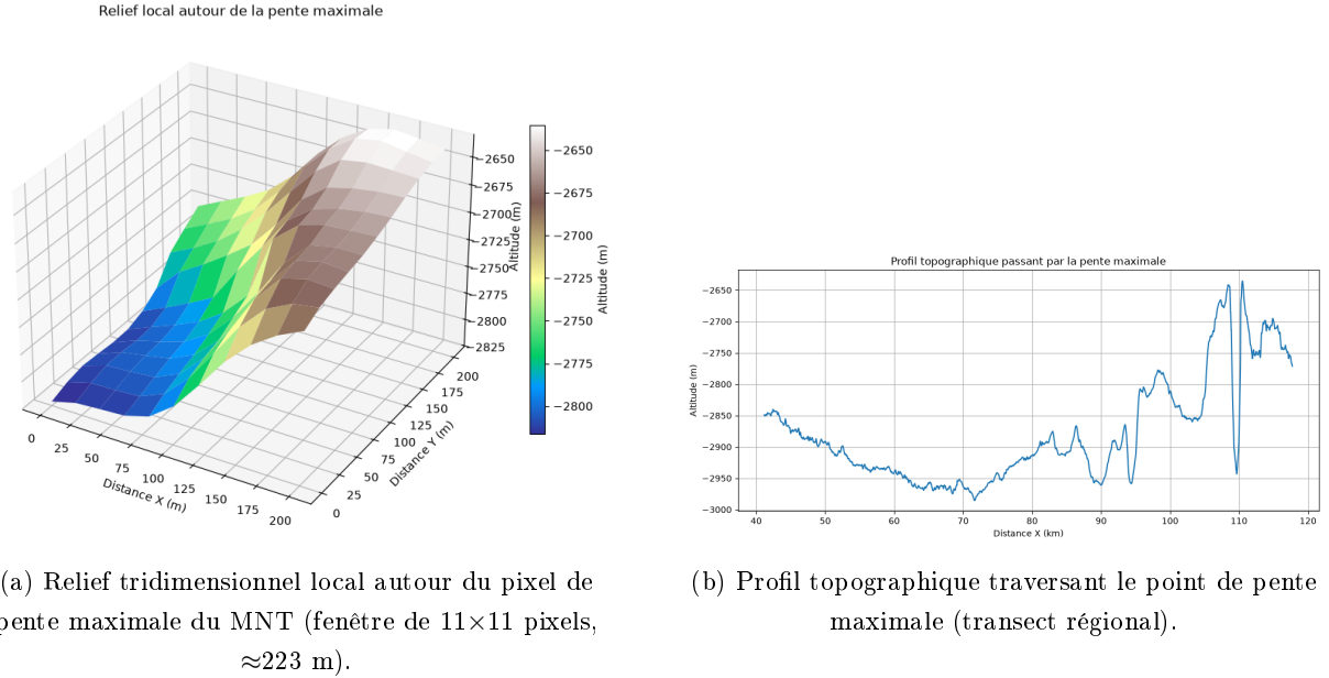
Figure 4: Relief local (a) et profil régional (b) au niveau du maximum global de pente.
