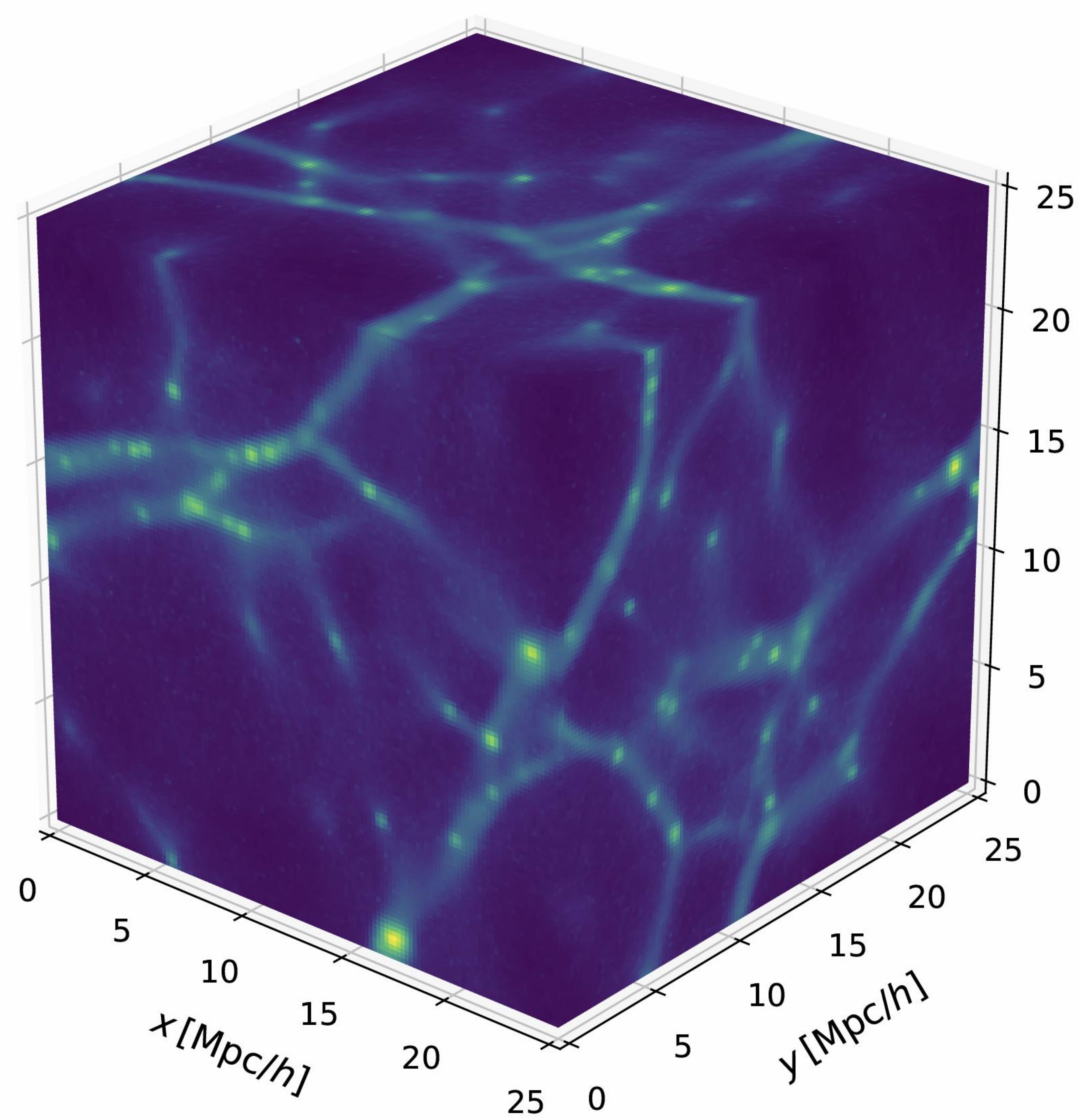
Posterior mean
