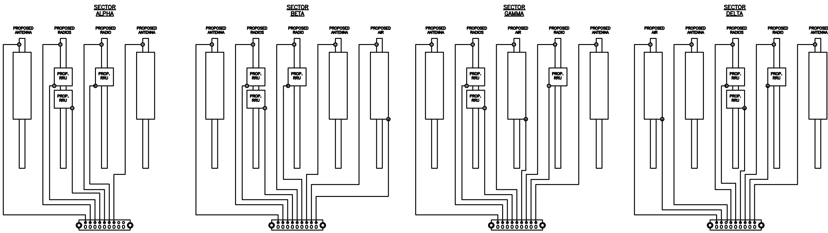
3 ANTENNA & RADIOS GROUNDING DIAGRAM SCALE: N.T.S
