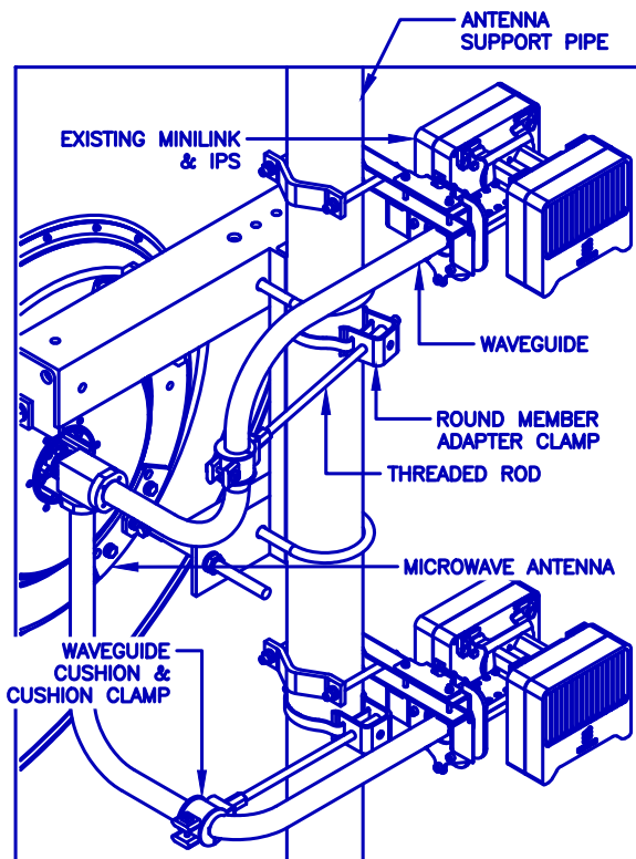
WAVEGUIDE CLAMP DETAIL SCALE: N.T.S
