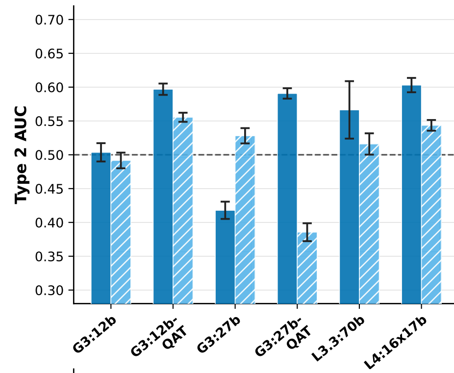
Type2 AUC
