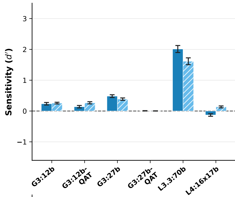
Sensitivity ( d' )
