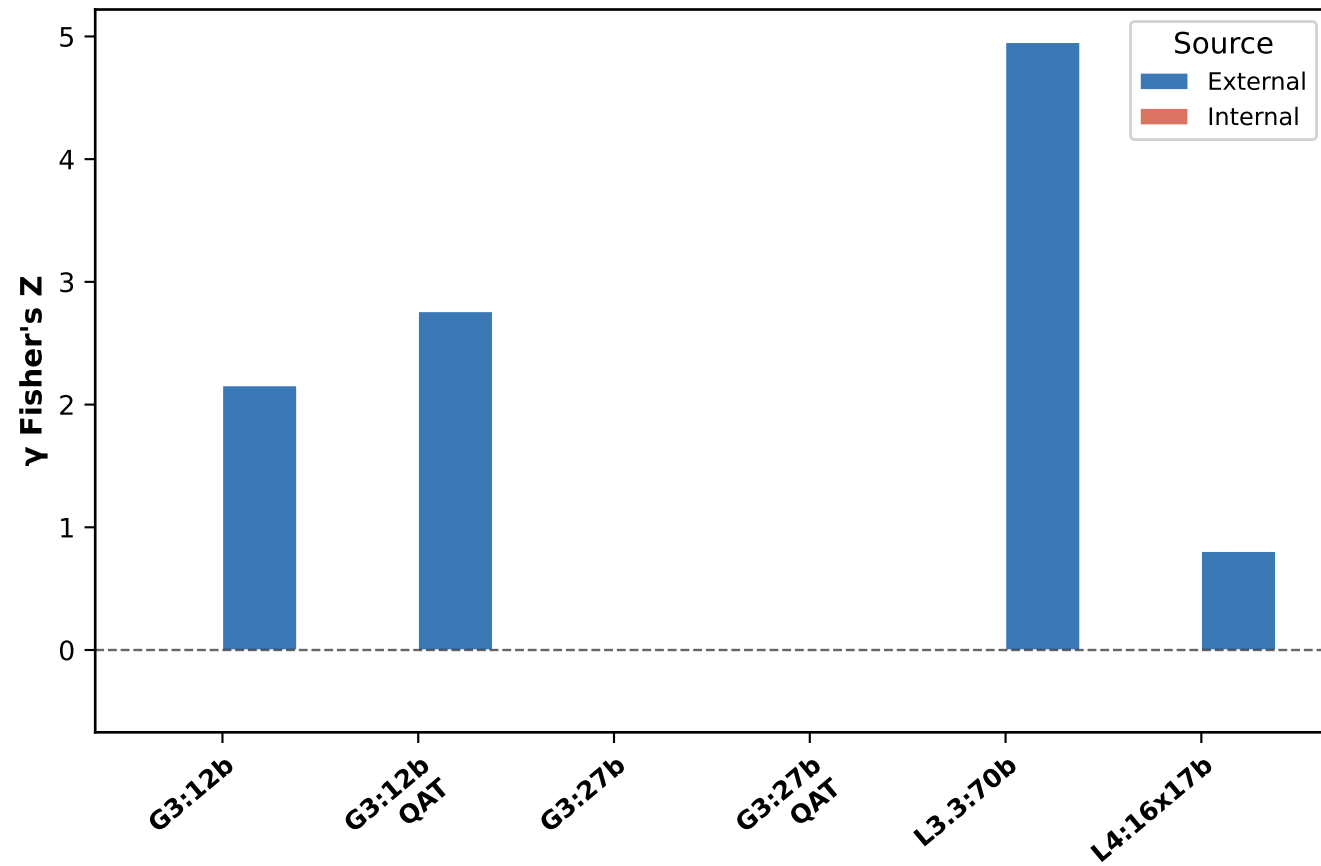
SingleTurn
