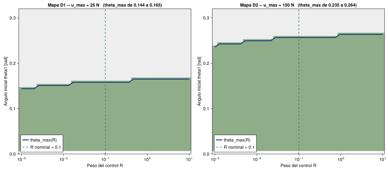
Figura 6: Ángulo recuperable en función del peso R del control, para un actuador limitado (izquierda) y uno holgado (derecha).
