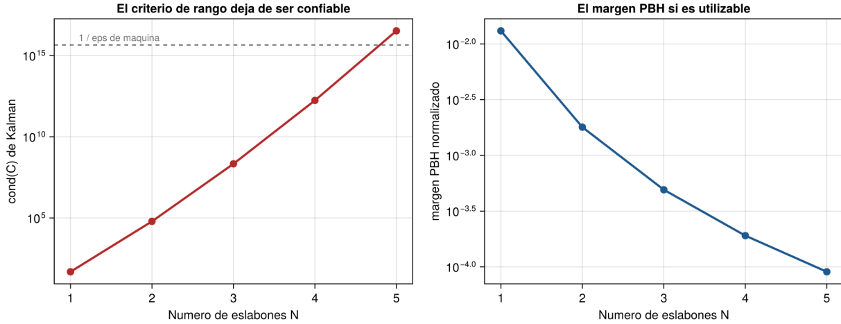
Figura 3: Izquierda: el condicionamiento de la matriz de Kalman crece catorce órdenes de magnitud entre N = 1 y N = 5 , cruzando el umbral de 1/\varepsilon_{\text{máq}} . Derecha: el margen PBH decae suavemente, apenas dos órdenes y medio, y sigue siendo utilizable.
