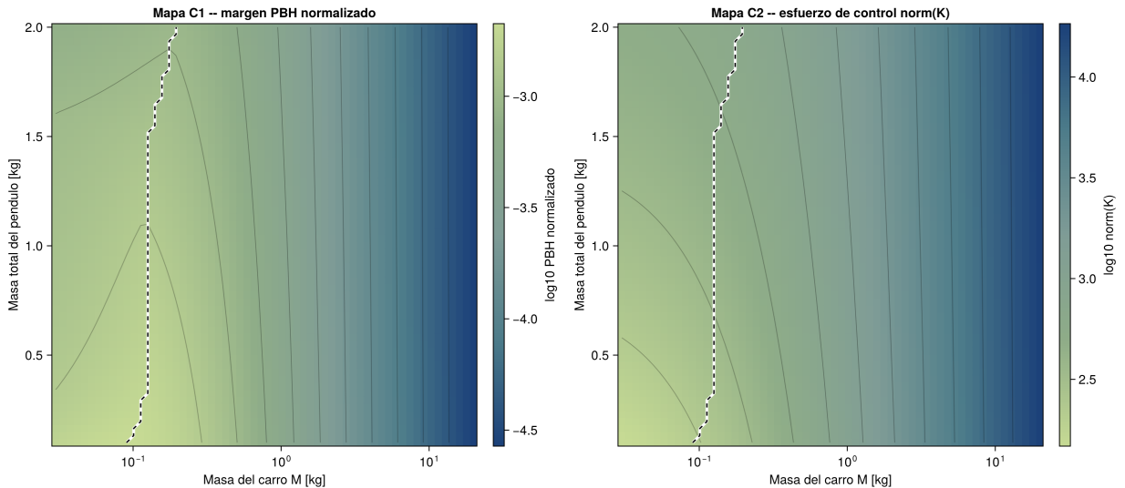
Figura 5: Mapa de la masa del carro contra la masa total del péndulo. La línea segmentada marca, para cada masa de péndulo, la masa de carro que maximiza el margen PBH. En ambos paneles el color claro es “mejor”. El óptimo del margen no coincide con el del esfuerzo de control, que es monótono.
