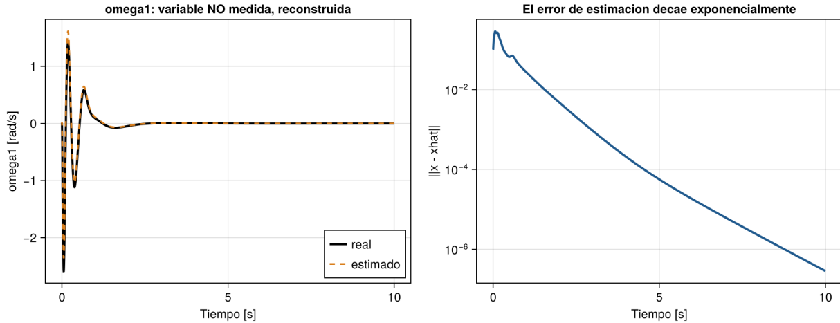
Figura 7: Izquierda: reconstrucción de \omega_1 , que no se mide, a partir de la posición y los tres ángulos. Derecha: el error de estimación decae exponencialmente —una recta en escala logarítmica— como predice \dot{e} = (A - LC)e con A - LC de Hurwitz. Condición inicial: \theta_1 = 0.10 rad con el estimador arrancando en cero.
