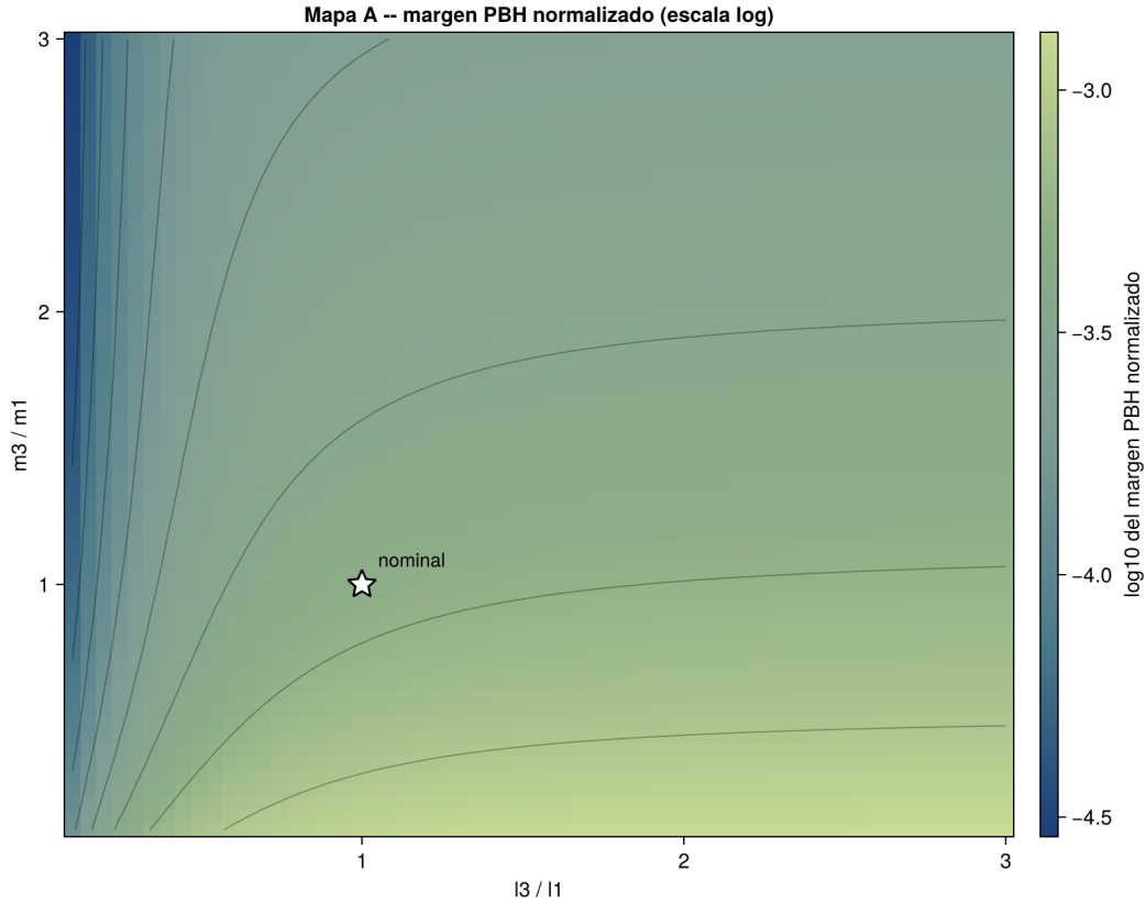
Figura 6: Región estructuralmente sana en el plano de las razones geométricas del eslabón superior. La estrella marca la configuración nominal ( l_3/l_1 = m_3/m_1 = 1 ). El margen es máximo abajo a la derecha: eslabón superior largo y ligero . Ambos efectos van en el mismo sentido, pero el de la longitud es el dominante: a masa nominal, pasar de l_3/l_1 = 0.1 a 3 multiplica el margen por 10.6, mientras que a longitud máxima, aligerar de m_3/m_1 = 3 a 0.1 lo multiplica por 5.0.
