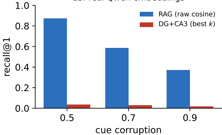
E3: real Qwen embeddings
