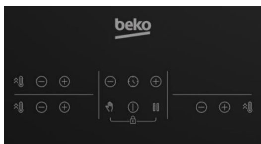
MIND
