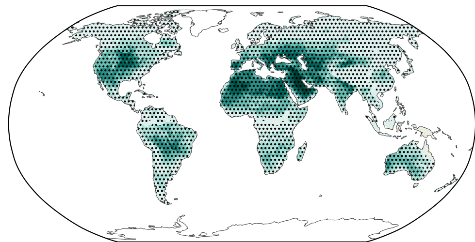
CESM2-WACCM G6-SAI – SSP2-4.5
