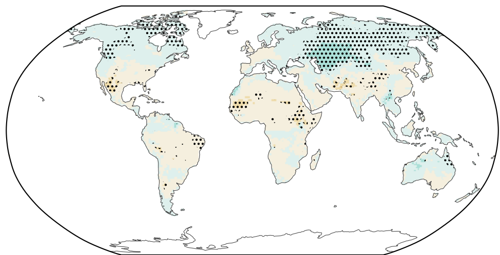
CESM2-WACCM G6-HiLLA – G6-SAI
