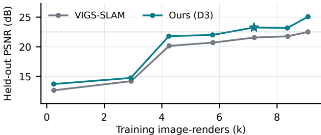
VIGS-SLAM
