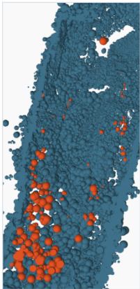
VIGS-SLAM
