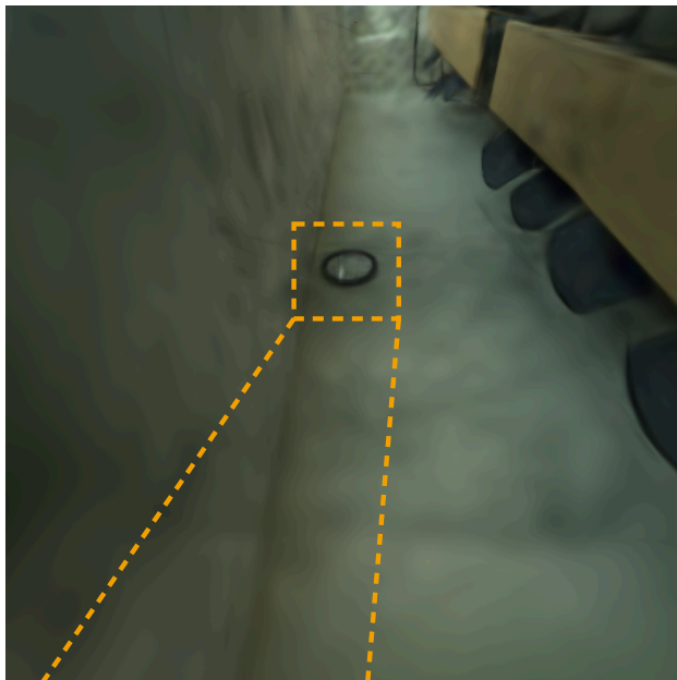
Ours
