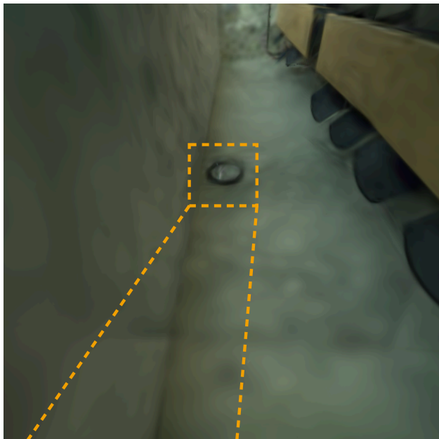
VIGS-SLAM
