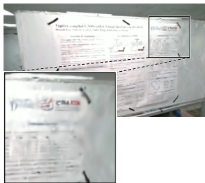
VIGS-SLAM
