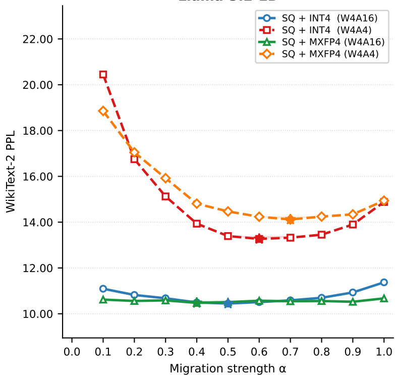
Llama-3.2-1B
