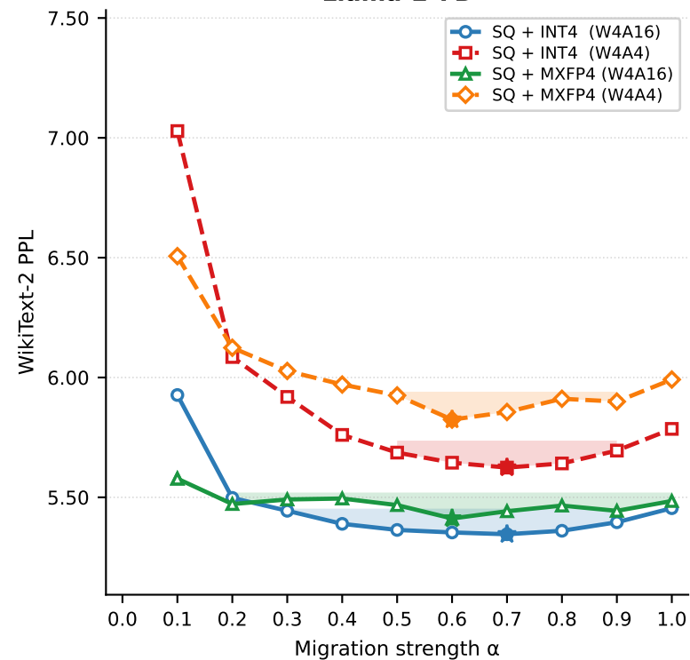
Llama-2-7B
