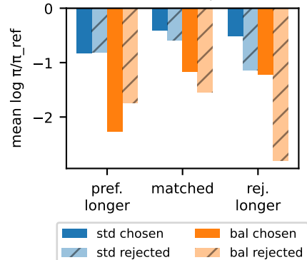
(d) Likelihood displacement
