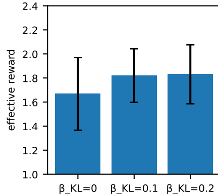
(d) KL forks: held-out reward
