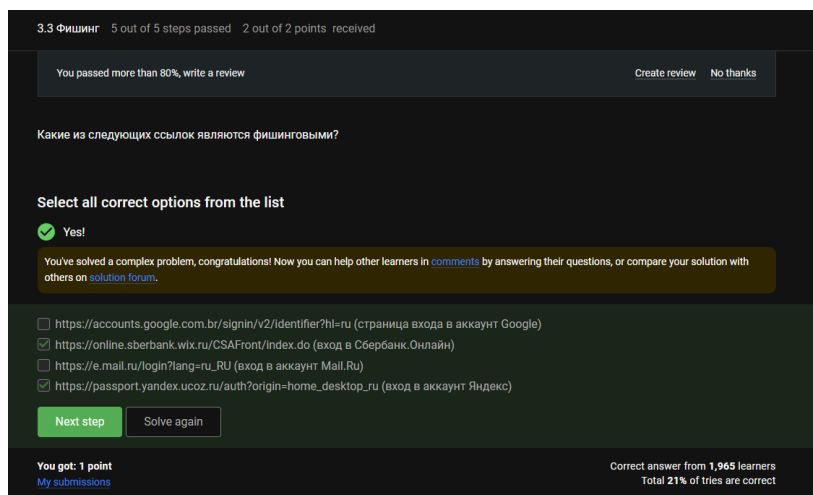
Рисунок 2.10: Фишинговая ссылка
