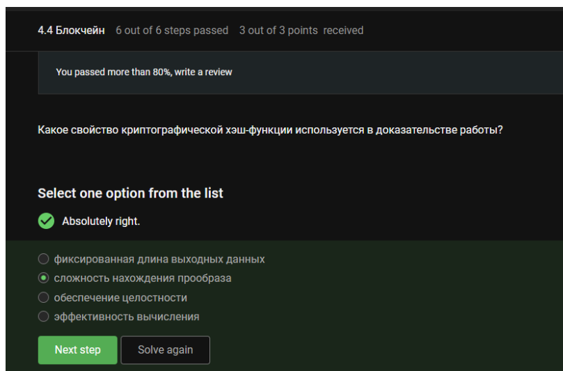
Рисунок 2.14: Криптографическая хэш-функция
