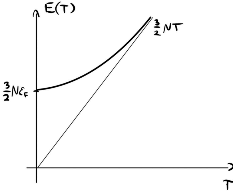
Рис. 1.2: Средняя энергия ферми-газа в зависимости от температуры.
