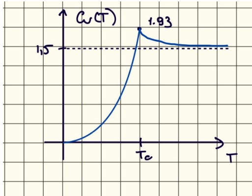
Рис. 1.3: Теплоёмкость идеального бозе-газа в зависимости от температуры. Излом в точке T_c — признак фазового перехода.
