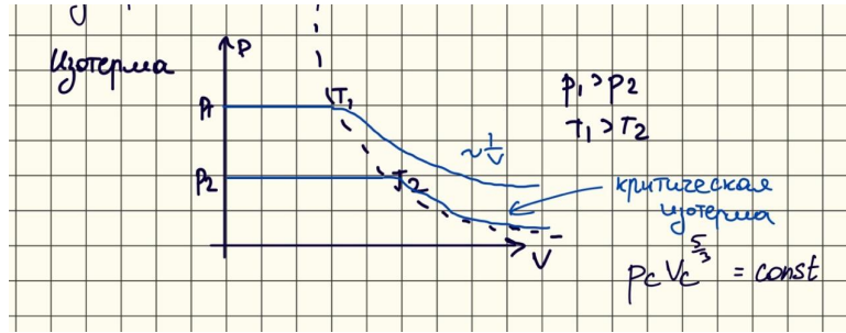
Рис. 1.4: Изотермы идеального бозе-газа. Горизонтальный участок соответствует области бозе-конденсации.
