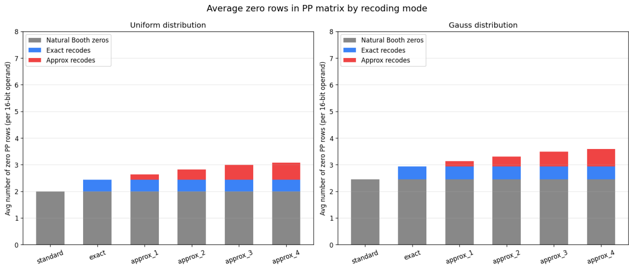
Рис. 4: Среднее число нулевых строк partial product матрицы (natural + exact recodes + approx recodes) по режимам recoding для двух распределений.
