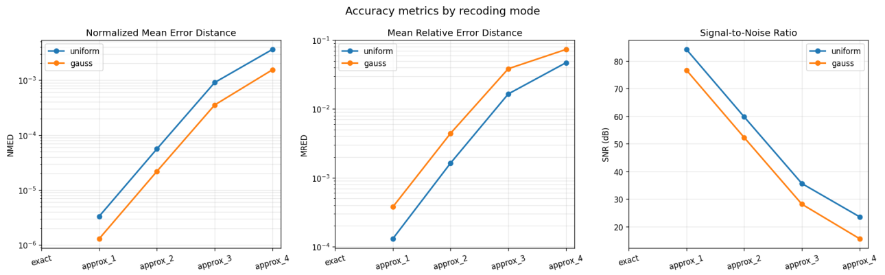
Рис. 3: NMED, MRED и SNR в зависимости от режима recoding для uniform и gauss распределений.
