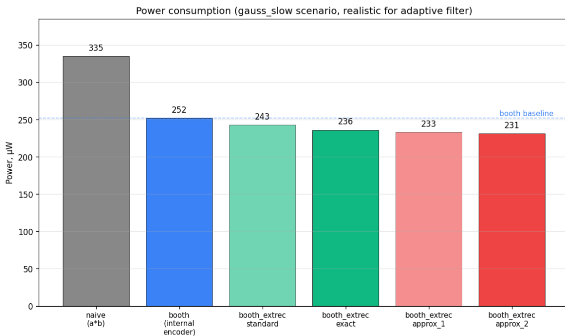
Рис. 1: Мощность всех конфигураций умножителя в сценарии gauss_slow.
