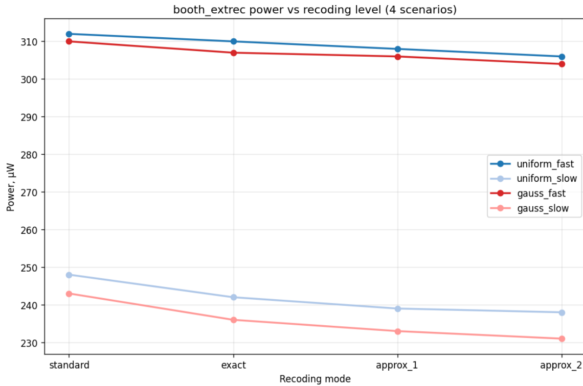
Рис. 2: Мощность booth_extrec в зависимости от режима recoding для четырёх сценариев стимулов.
