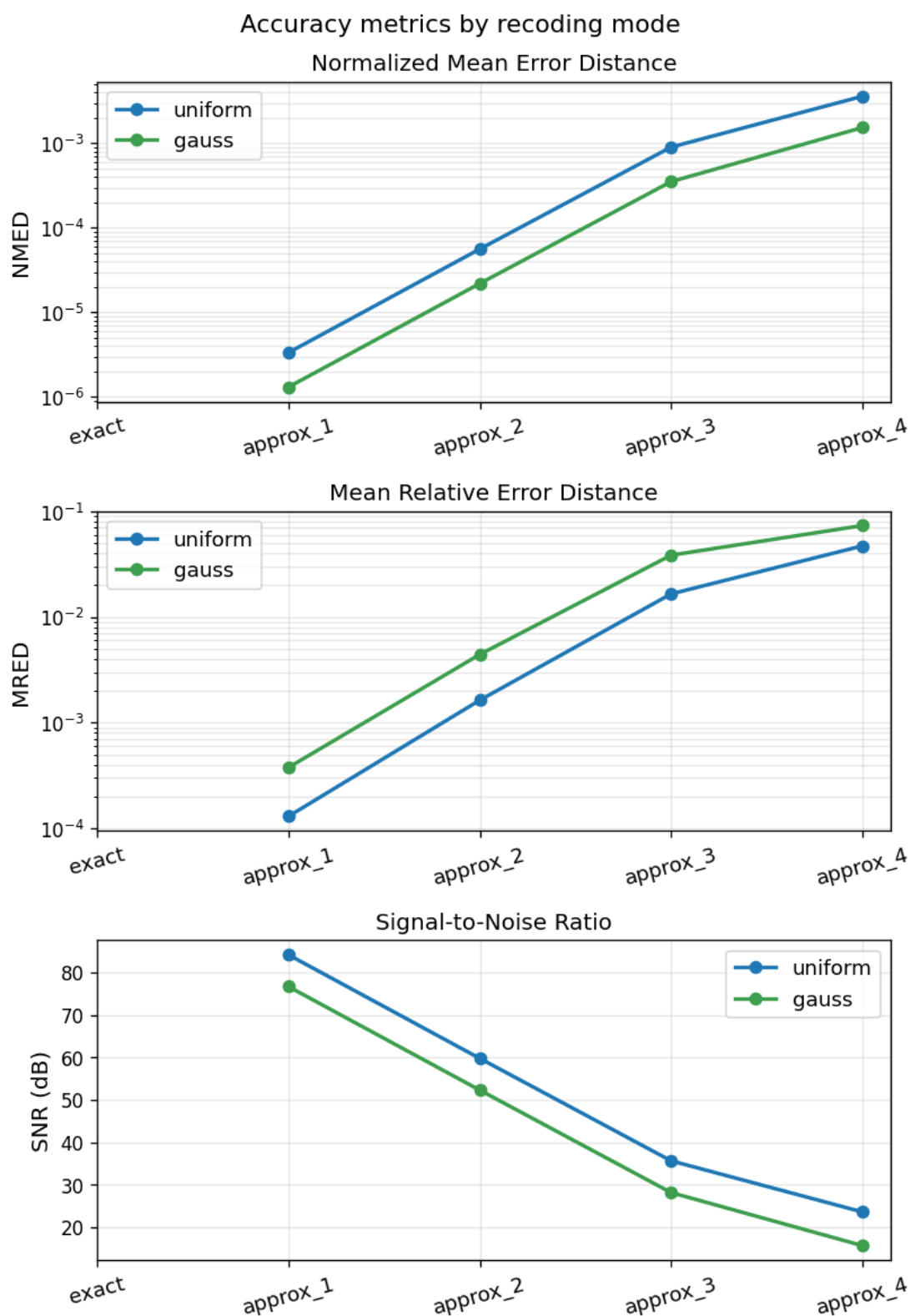
Рисунок 10 — Метрики точности по режимам перекодировки: NMED, MRED, SNR (кривые для равномерного и гауссового распределений)
