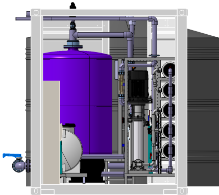
RIGHT WIEW
