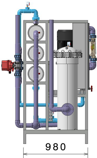
Vue de gauche
