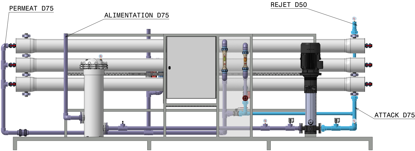
Vue de face
