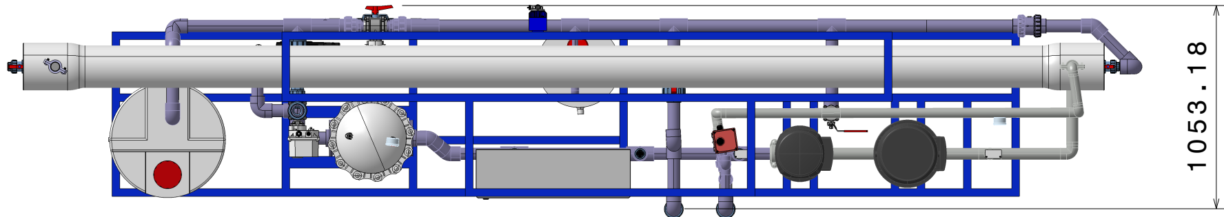
Vue de dessus
