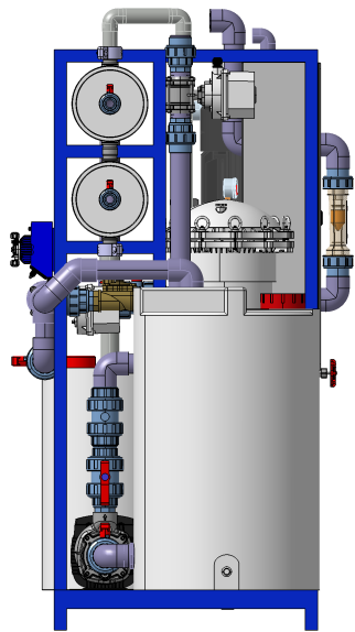
Vue de gauche
