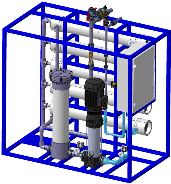
Vue isométrique
