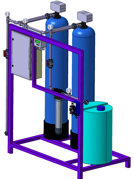
Vue isométrique
