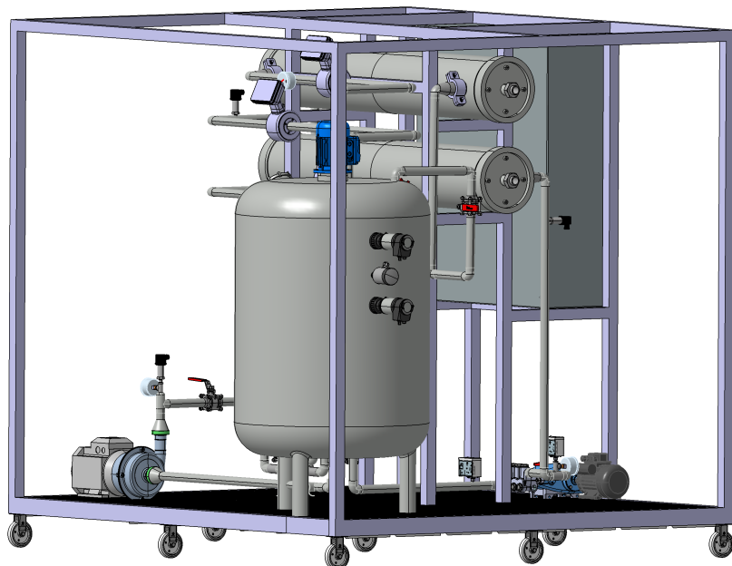
Vue isométrique
