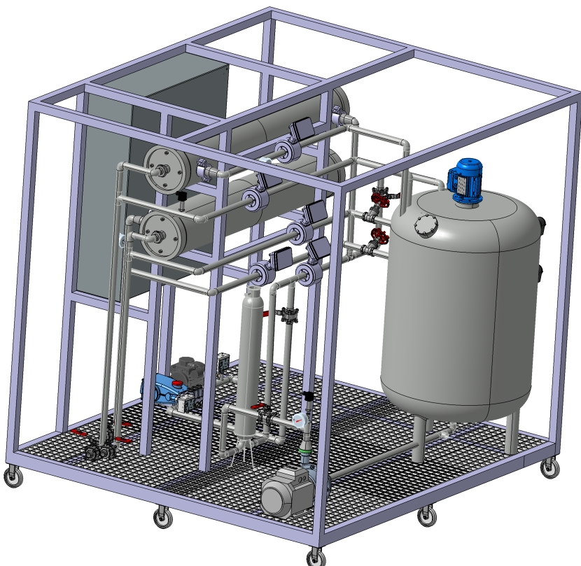
Vue isométrique
