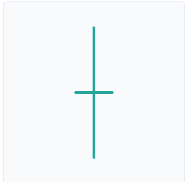
Doji
