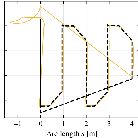
PPO
