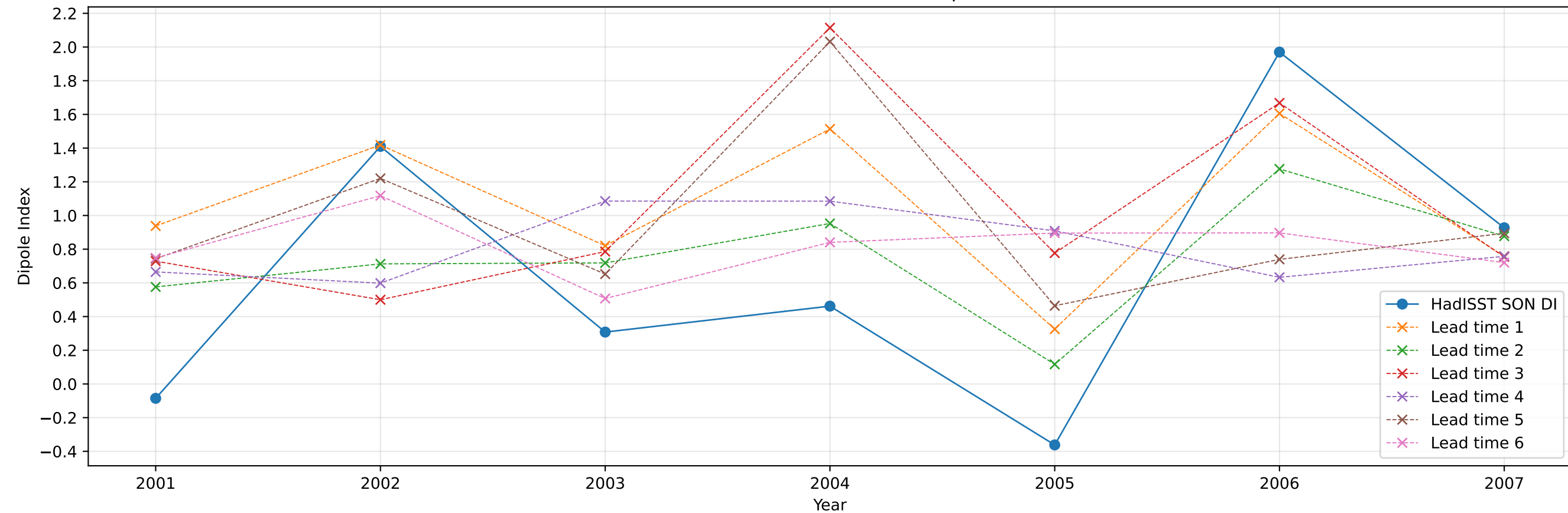
SON DI: HadISST vs CNN ensemble prediction
