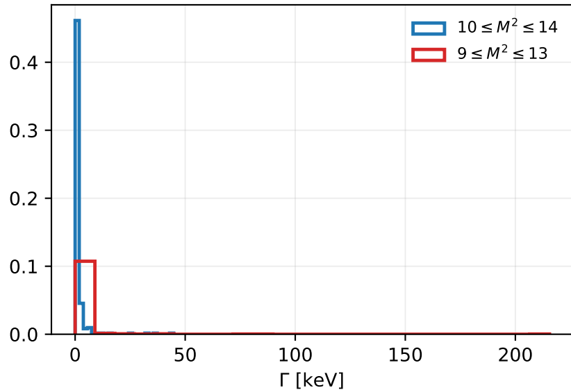
B_{s1}(5830)
