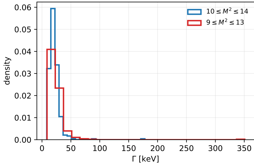
B_{s1}(5750)
