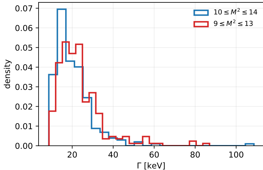
B_{s1}(5750)
