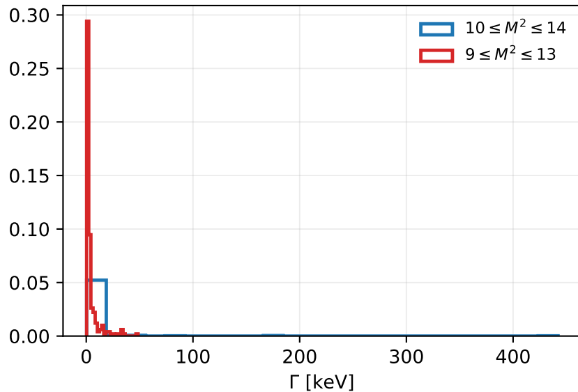
B_{s1}(5830)
