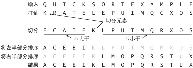
图 2.3.1 快速排序示意图
