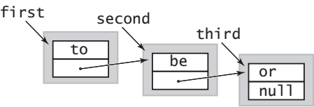
图 1.3.5 用链接构造一条链表
