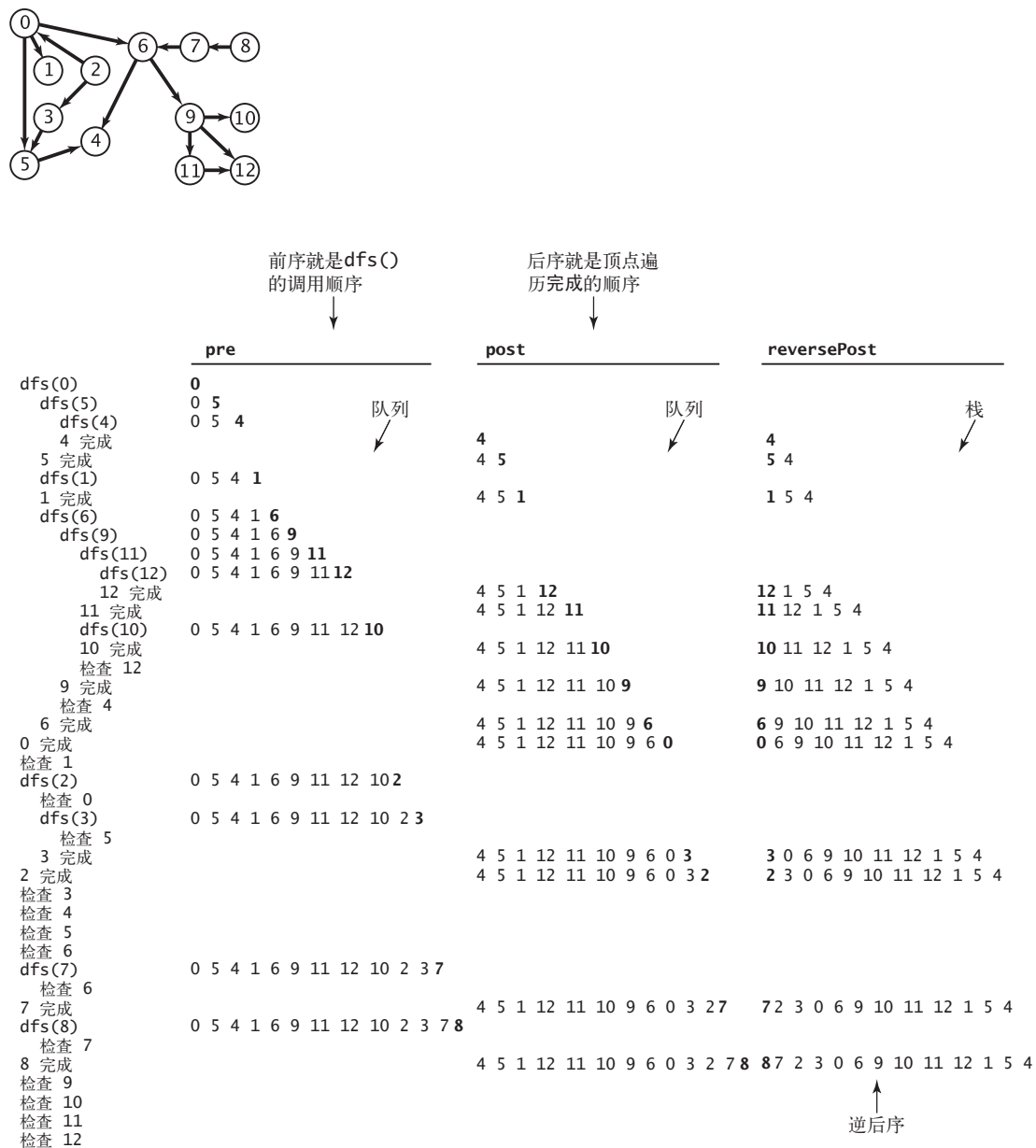
579 图 4.2.10 计算有向图中顶点的深度优先次序（前序、后序和逆后序）
