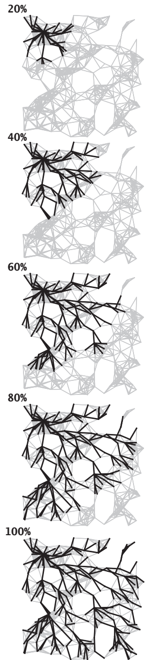
图 4.1.20 使用广度优先搜索查找最短路径（250 个顶点）
