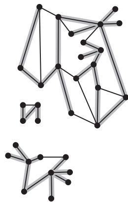
图 4.1.5 生成树森林
