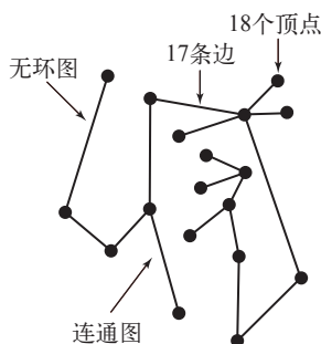
图 4.1.4 一棵树
