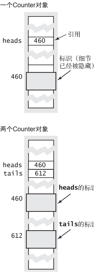
图 1.2.1 对象的表示
