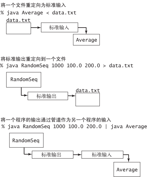
图 1.1.5 命令行的重定向与管道
