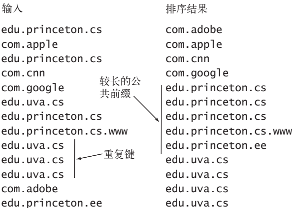
图 5.1.15 三向字符串快速排序的示意图 图 5.1.16 适于使用三向字符串快速排序的典型情况
