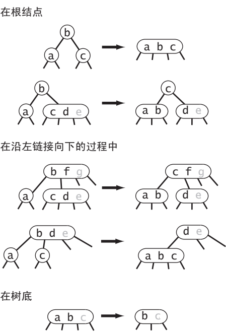
图 3.3.26 删除最小键操作中的变换
