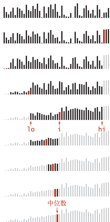
图 2.5.2 用切分找出中位数
