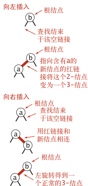
图 3.3.18 向单个 2- 结点中插入一个新键
