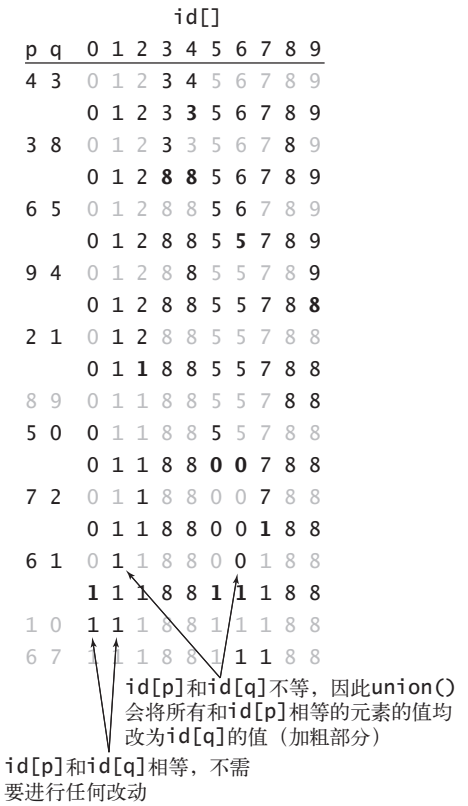
图 1.5.3 quick-find 的轨迹
