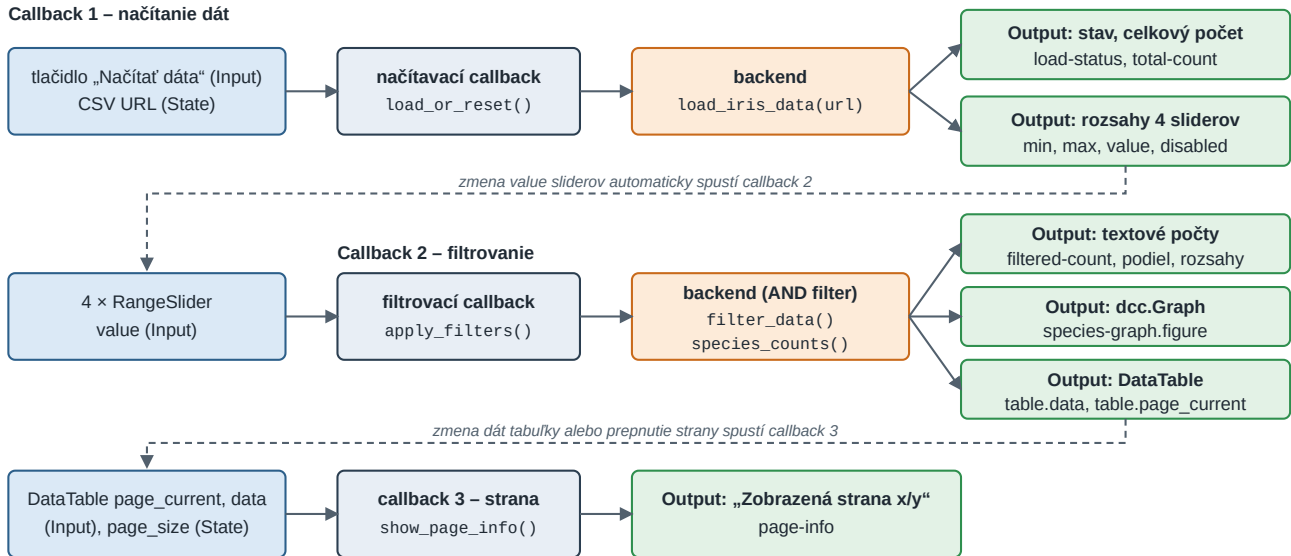
Obr. 5: Tok dát. Modré bloky sú vstupy (Input/State), sivé callbacky, oranžové backend, zelené výstupy (Output). Prerušované šípky ukazujú reťazenie: výstup jedného callbacku je vstupom ďalšieho.
